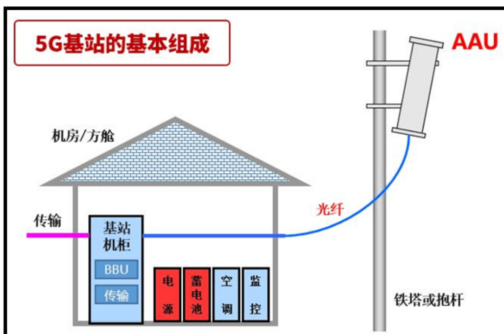
图 2-7 5G 基站的基本组成
